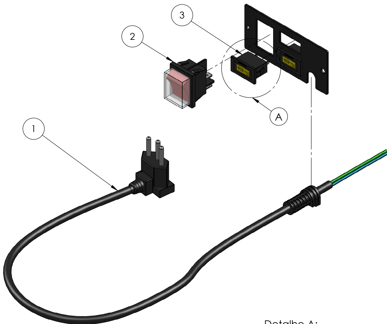
Detalhe A:
