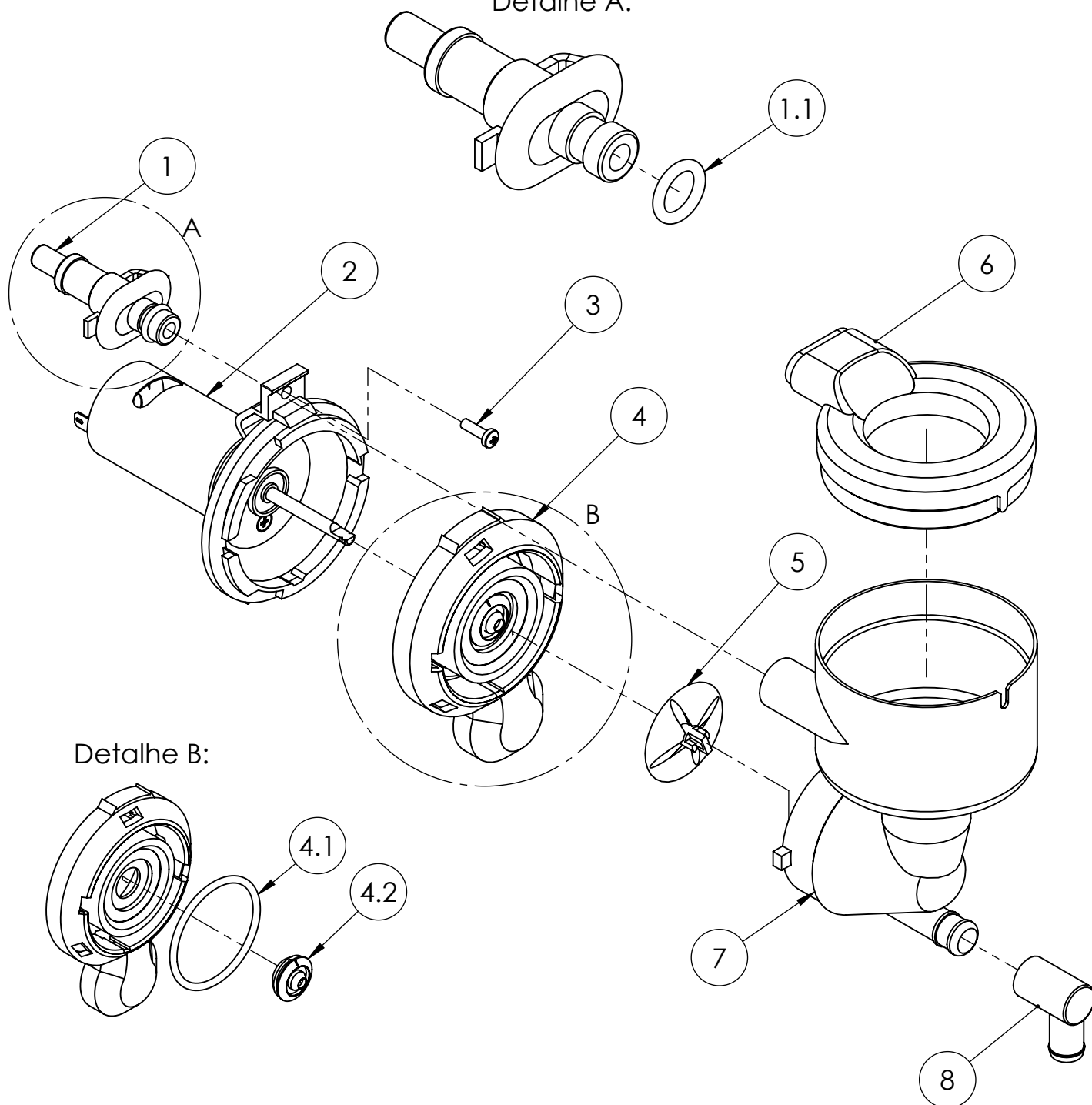
Detalhe A:
